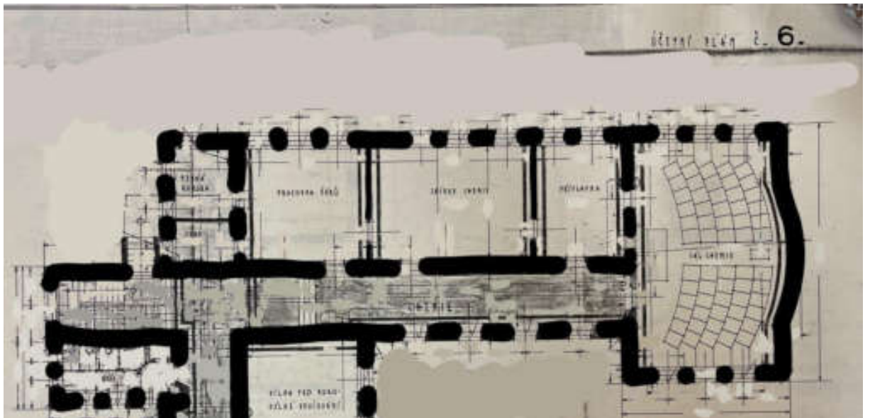
[obr. 8] HERYNK, Rudolf. Účetní plán č. 6: Souterrain [půdorys]. Měřítko 1:100. [1924]. Archiv stavebního úřadu v Brandýse nad Labem – Stará Boleslavi. Veřejně nepřístupný dokument.
