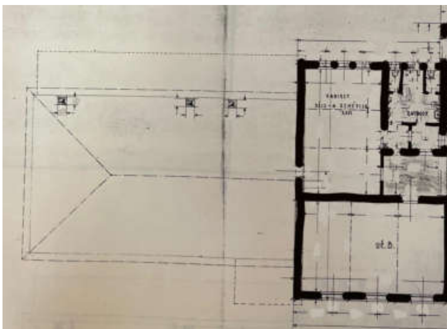
[obr. 6] HERYNK, Rudolf. Účetní plán č. 9: II. patro [půdorys]. Měřítko 1:100. [1924]. Archiv stavebního úřadu v Brandýse nad Labem – Stará Boleslavi. Veřejně nepřístupný dokument.
