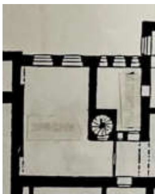
[obr. 5] VALEČKA, Jaroslav. Plány nové školní budovy: Suterén [půdorys]. Měřítko 1:20. Praha, [1924]. Gymnázium J. S. Machara Brandýs nad Labem – Stará Boleslav. Veřejně nepřístupný dokument.
