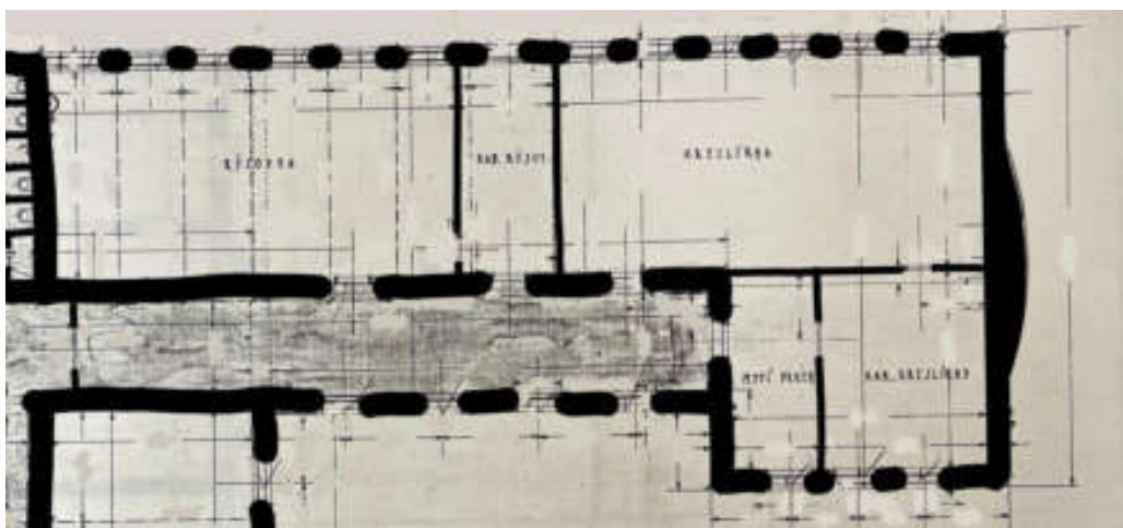
[obr. 7] HERYNK, Rudolf. Účetní plán č. 8: I. patro [půdorys]. Měřítko 1:100. [1924]. Archiv stavebního úřadu v Brandýse nad Labem – Stará Boleslavi. Veřejně nepřístupný dokument.
